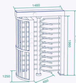
Technický výkres DS411 – rozmery
